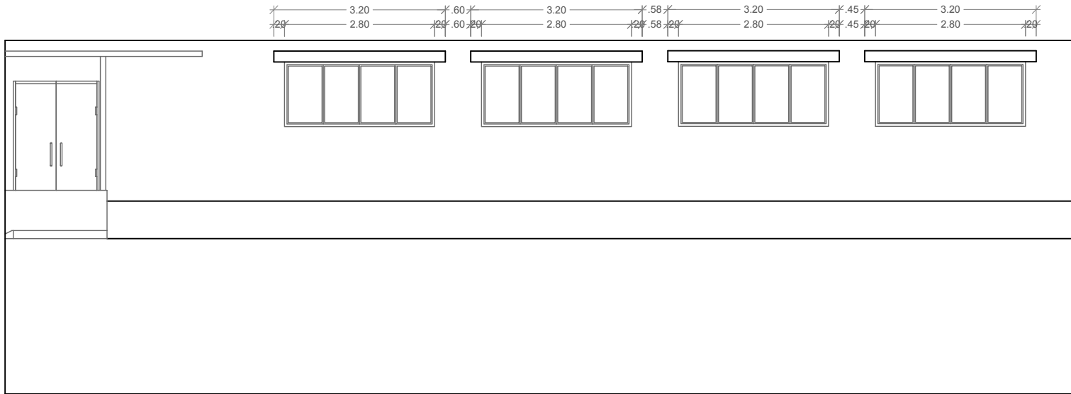
1 ELEVACION FRONTAL FACHADA/TOLDOS A-1 ESC. 1:100
